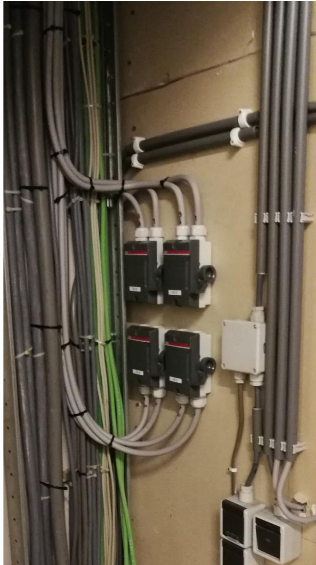
4 schakelaars Per dimmergroep een schakelaar
